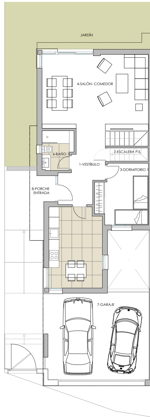
PLANTA BAJA sin escala
